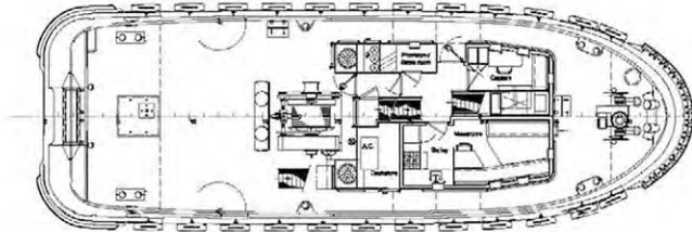
Maindeck
